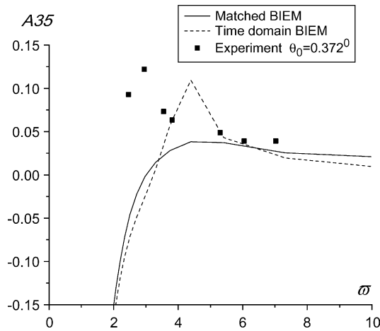
Fig. 23. F_n=0.3 .
