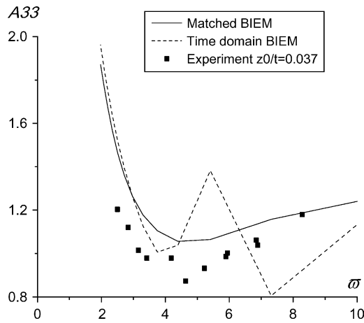
Fig. 19. F_n=0.3 .
